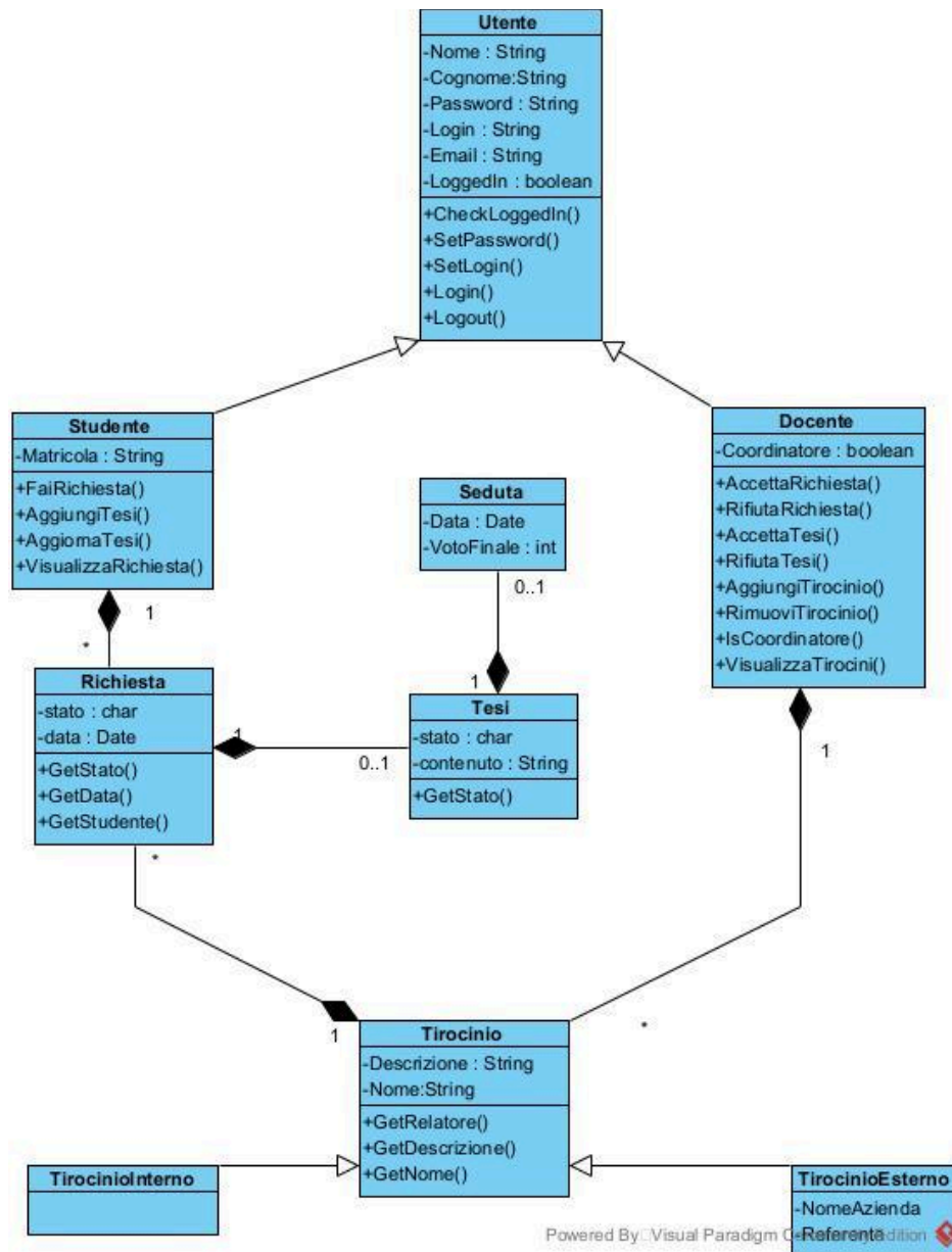
Immagine 1 Class Diagram in Universal Modeling Language (UML)
